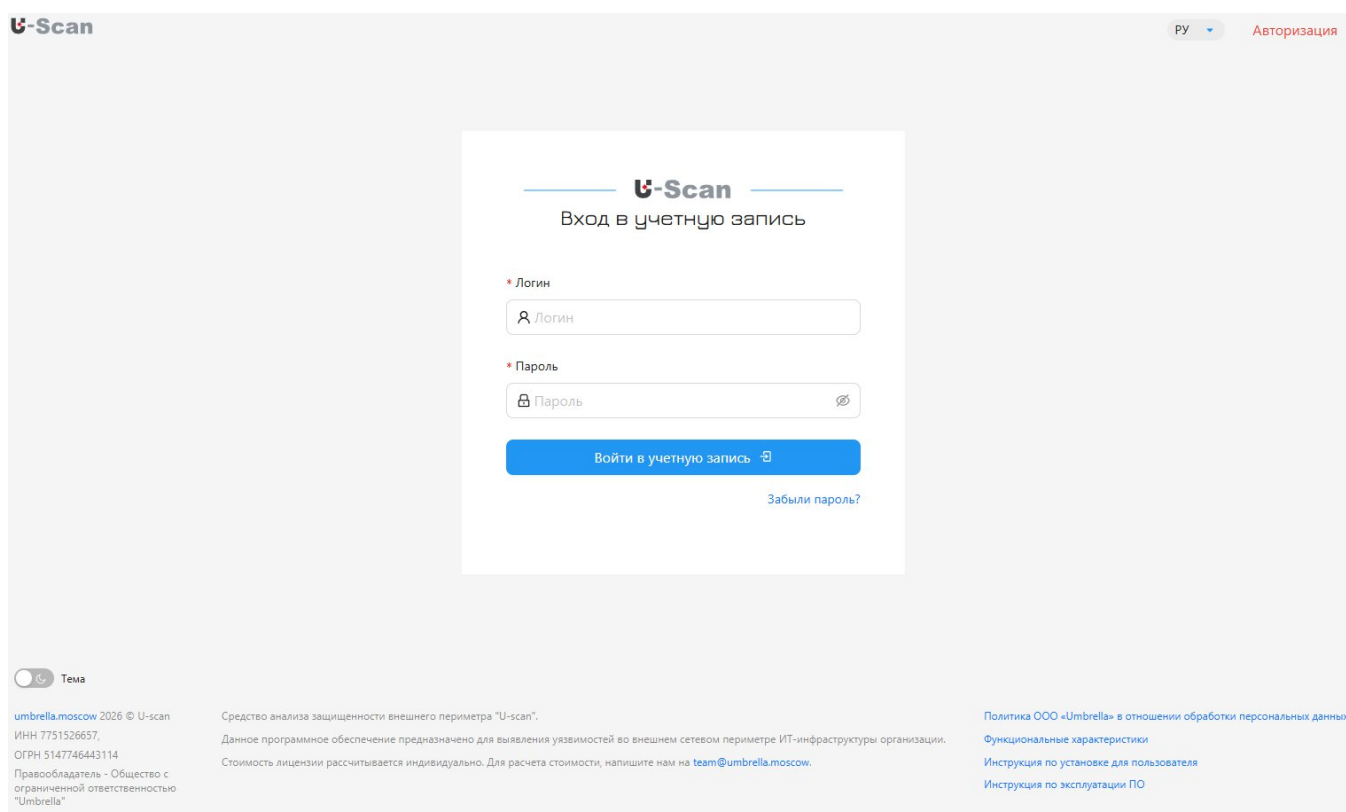
Рисунок 1 – Начальная страница
